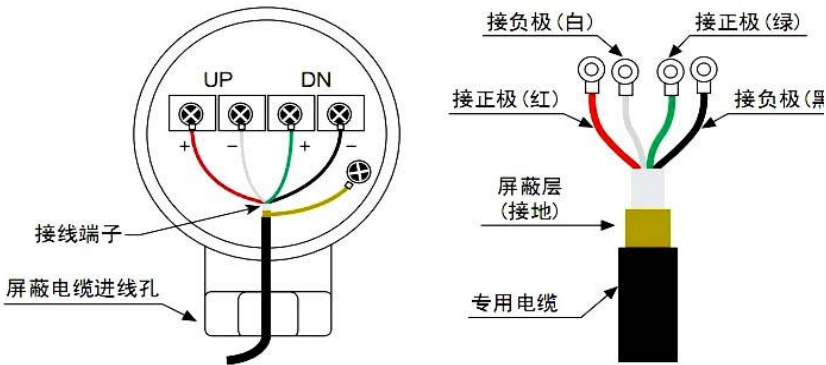
传感器接线图
