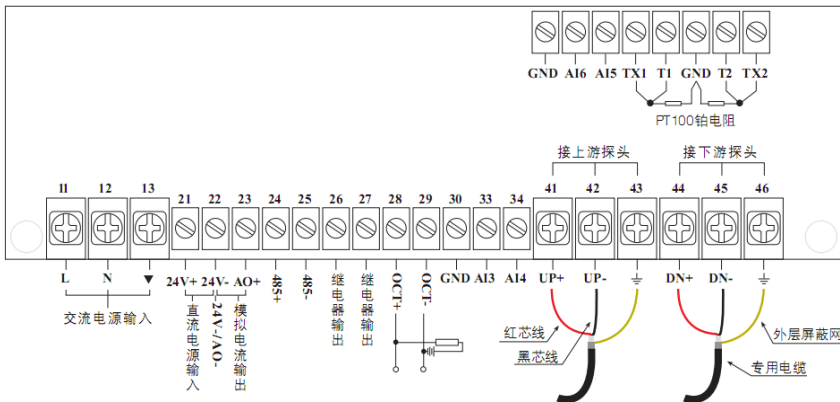
15 版本板接线图
