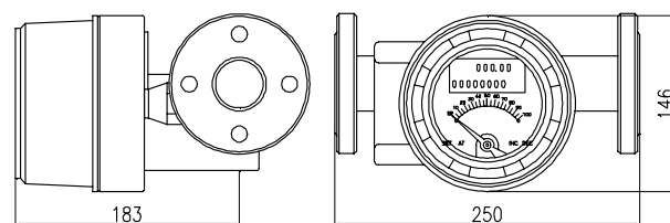
图 11 弹簧结构 M5 指示器
