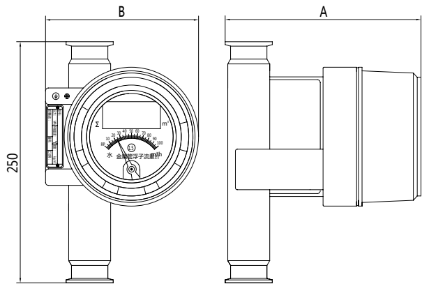
图7 卫生型 M5 指示器
