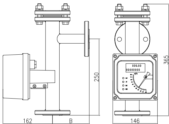
图 12 标准型 M4 指示器
