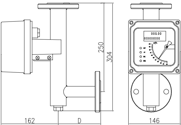
图 16 标准型 M4 指示器
