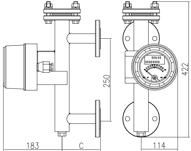
图 15 标准型 M5 指示器
