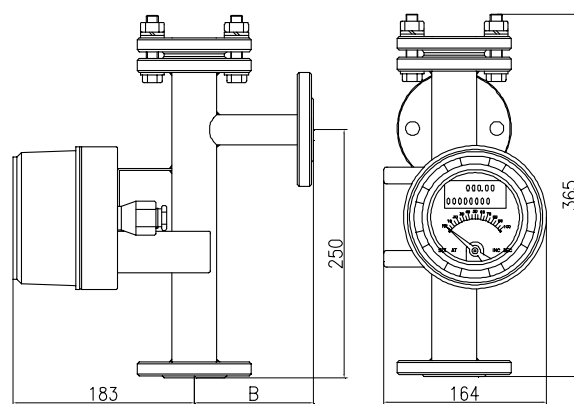
图 13 标准型 M5 指示器
