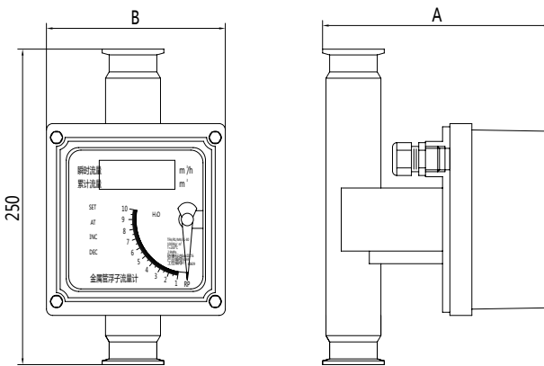
图6 卫生型 M4 指示器
