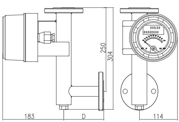
图 17 标准型 M5 指示器
