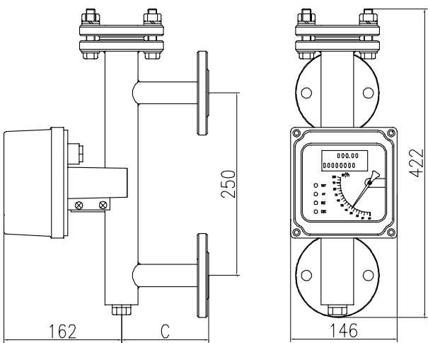
图 14 标准型 M4 指示器
