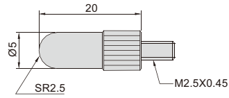
壳型测头
