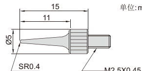
针测头
