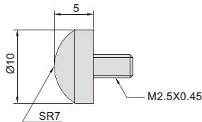
球面测头
