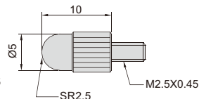
壳型测头
