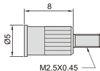
平测头
