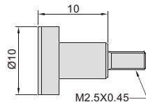
平测头
