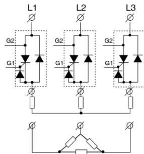
K9 三相三线半控功率模 块星型、三角型接线图 (单向可控硅+二极管)
