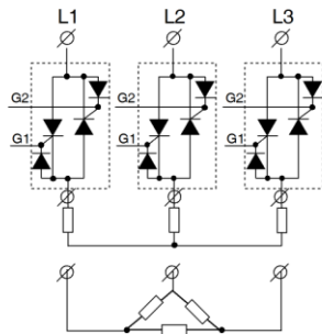
K9 三相三线全控功率模 块星型、三角型接线图 (单相可控硅反并联)
