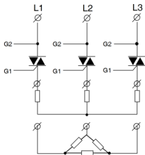
K9 三相三线星型、 三角型接线图 (双向 可控硅)
