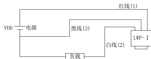
图 8-2 LWF- I 型前置放大器接线图
