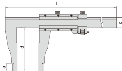
分体游尺
