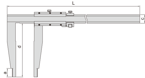
分体游尺
