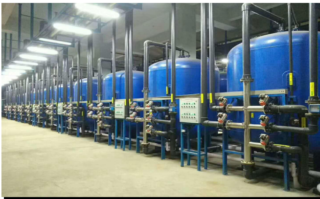
多介质过滤器
