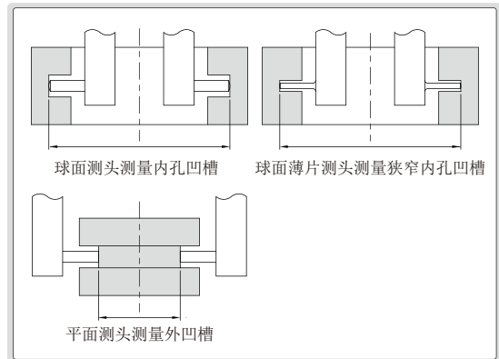
测量内凹槽和外凹槽
