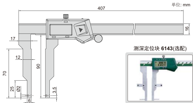
测量内凹槽和外凹槽
