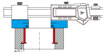
圆弧测量面测量孔内凹槽直径 (凹槽深度 h_2 \leq 7.5\text{mm} )
