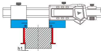
平面测量面测量外凹槽直径 (凹槽深度 h_1 \leq 2.5\text{mm} )
