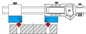
测量孔中心距
