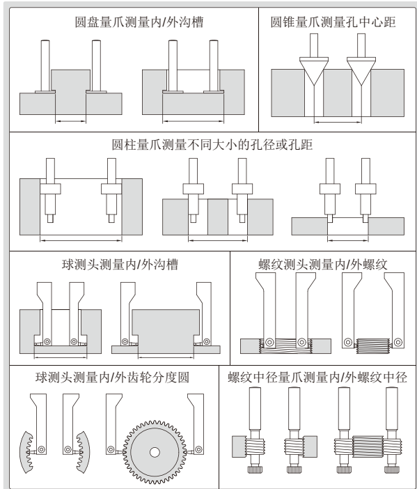
型号 1197-T501
