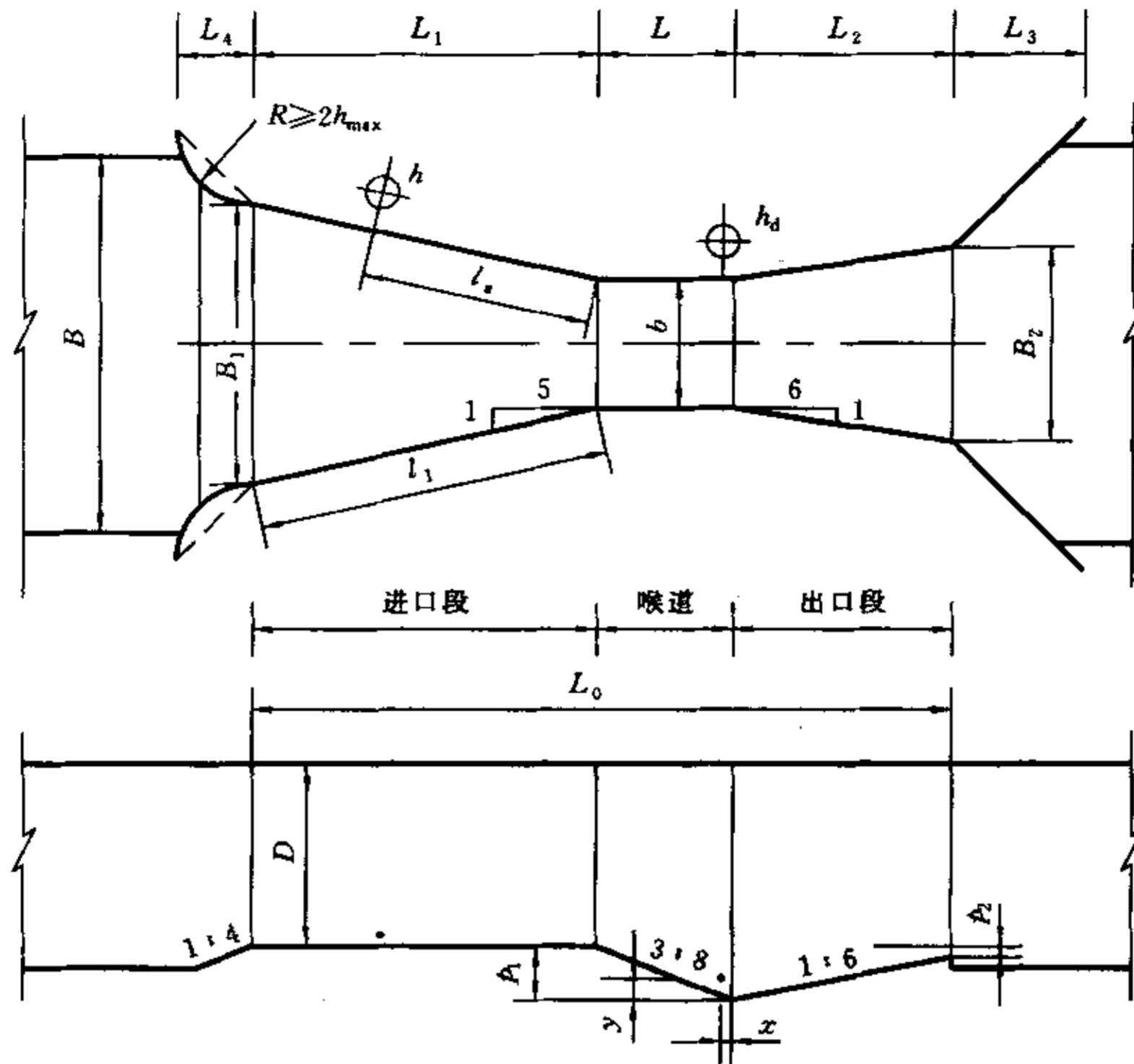
L —喉道长度; L —量水槽总长; L_1 —进口段轴线长度; L_2 —出口段轴线长度; L_3 —出口段护墙轴线长; L_A —进口段护墙轴线长; l_s —上游水头观测点到槽脊的距离; l_1 —进口段侧壁长; b —喉道宽; B —上游渠道宽; B_1 —进口段上游底宽; B_2 —出口段下游底宽; h —上游水头; h_d —下游水头; h_{max} —上游最大水头; R —进口护墙的曲率半径; p_1 —槽脊高度; p_2 —出口段末端至脊顶的高度; x —下游观测孔与槽底的高差; y —下游观测孔与槽底的水平距离; D —边墙高度
