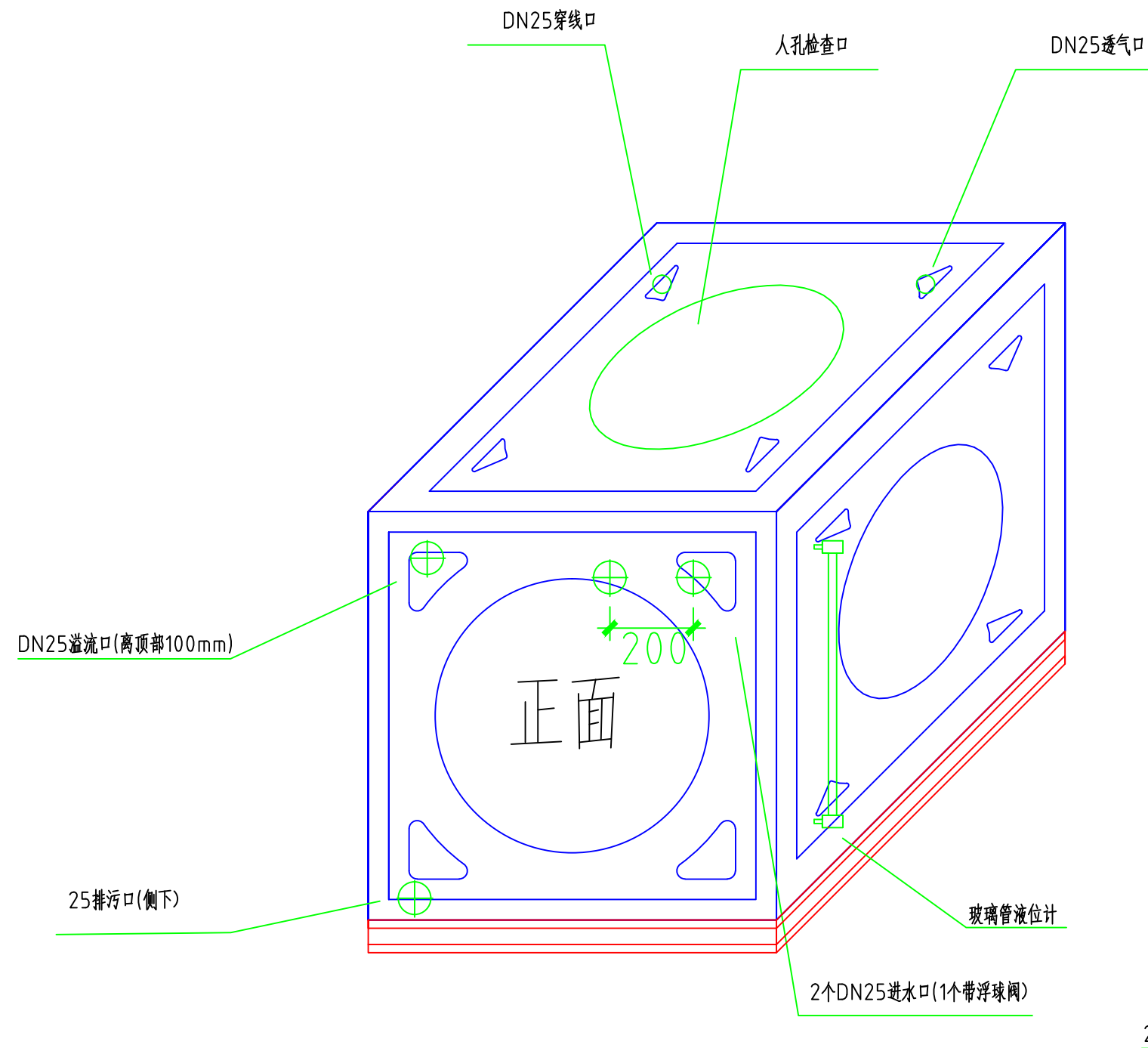
1×1×1(米) 保温水箱图
