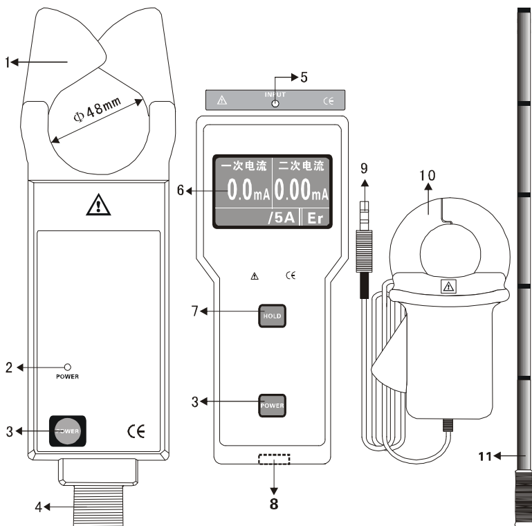
高压检测仪
