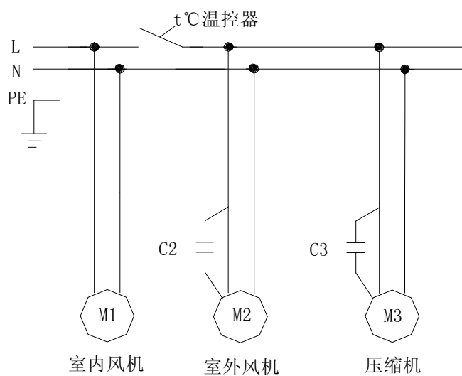
WEA-500Q 电路图
