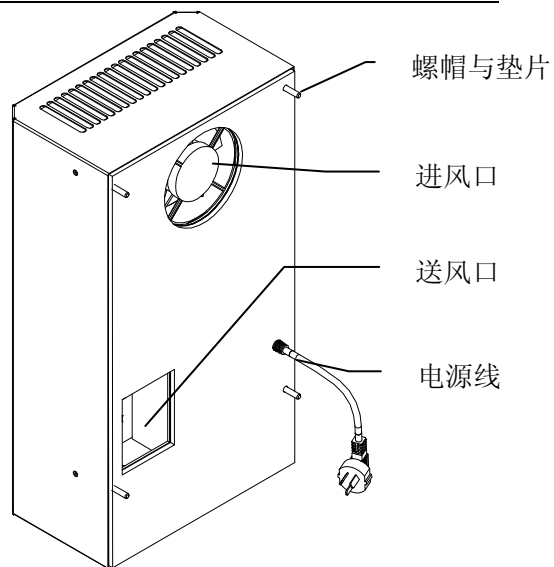
b. 卸下机组背后安装螺钉上的螺帽与垫圈，控制好螺栓的伸出长度约 15mm
