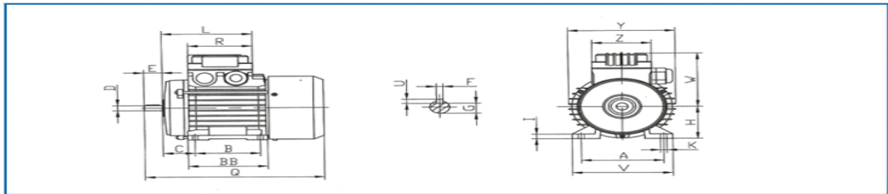
YS56尺寸 / YS56 DIMENSIONS
