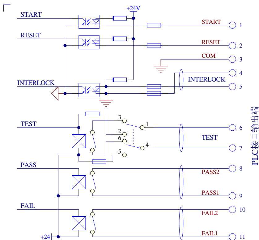
A: 仪器内部电路结构
