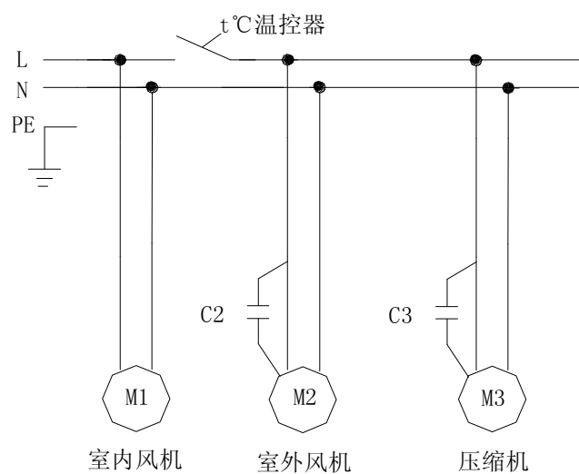
EA-450 电气原理图
