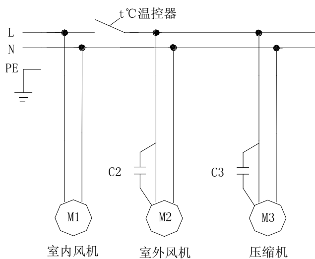
EA-600 电气原理图
