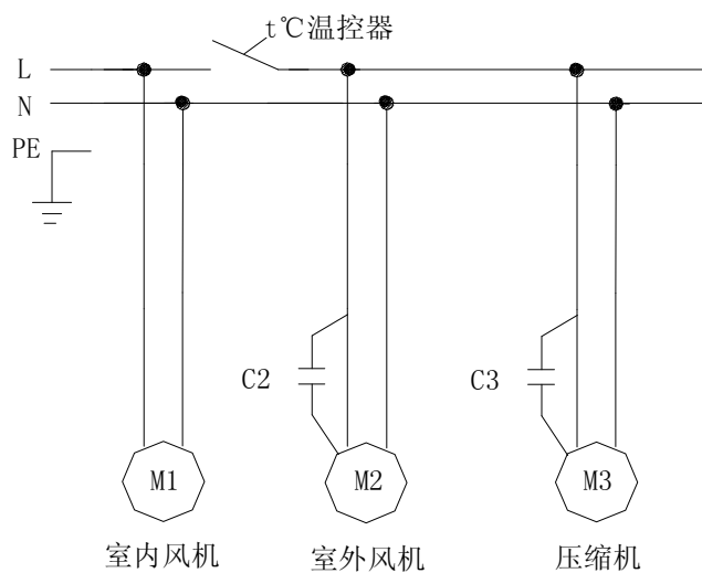
EA-800 电气原理图
