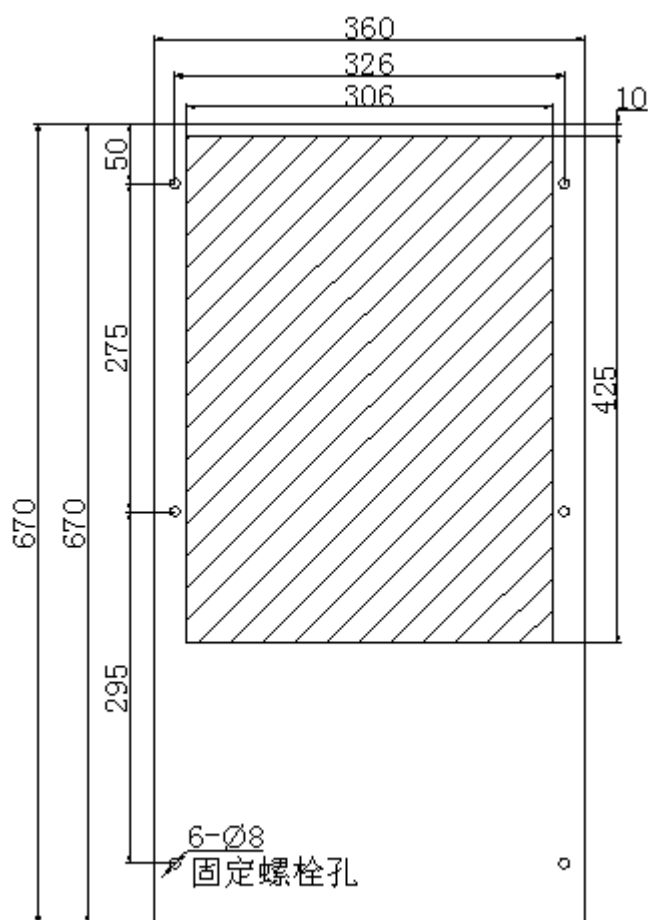
EA1000(阴影部分开孔 )
