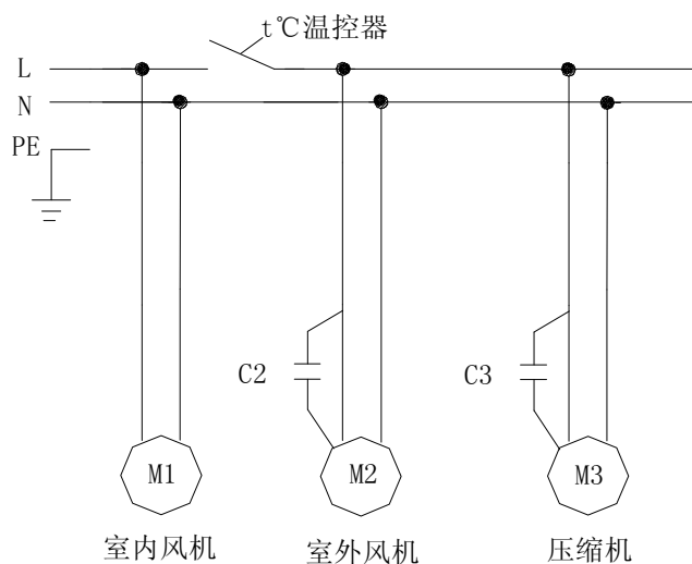
EA-1000 电气原理图
