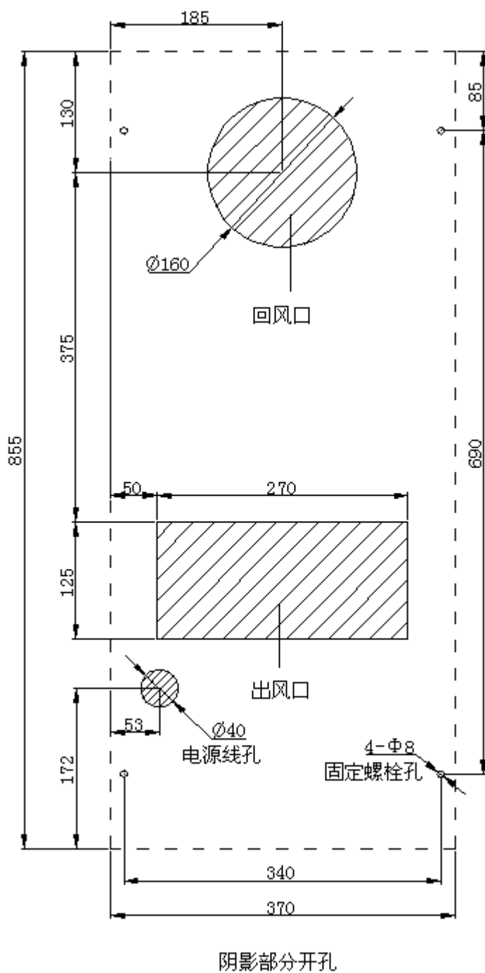
EA500(阴影部分开孔 )
